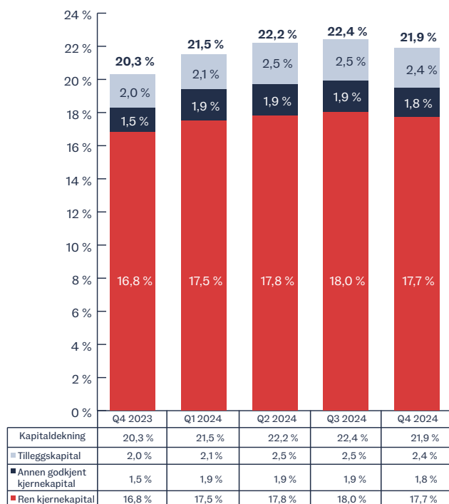
FIGUR 4: KAPITALDEKNING
